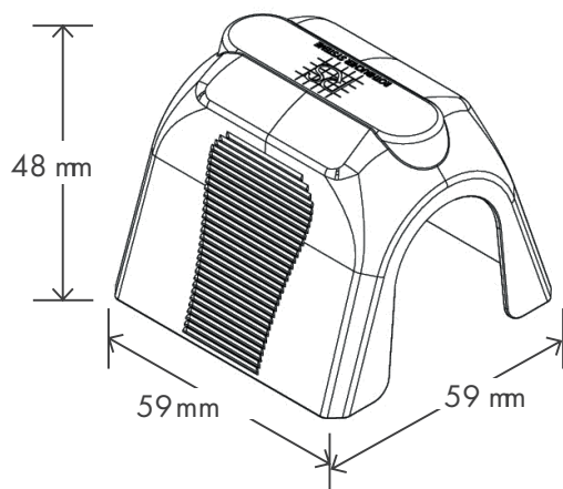
Schutzkappe RSPC20(M) Protection Cap RSPC20(M)
