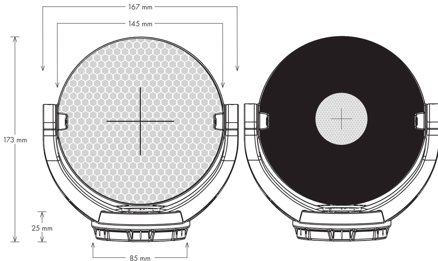
RSL452M Vorder/Rückseite – Front/Back RSL453M Vorderseite – Front
